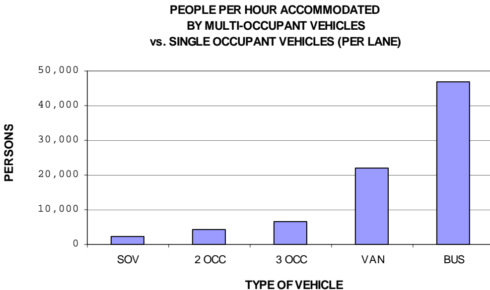
Figure 19. Persons per Hour per Travel Lane
